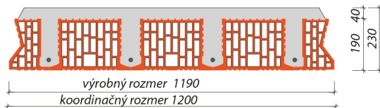
Základný rad – priečny rez panelmi šírky 1200, 900 a 600 mm
