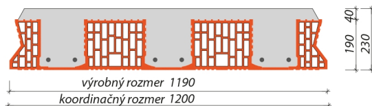
Panely PZU a balkónové – priečny rez panelmi šírky 1200 mm
