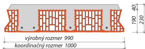
Doplňkový rad – priečny rez panelmi šírky 1000 a 700 mm
